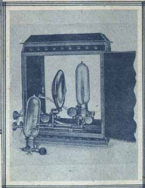
LANTERNA "SIMPLEX", COM LAMPADA INCANDESCENTE. AS VANTAGENS DESTE PROCESSO SOBRE O DO CARVÃO, É UM ASSUMPTO MUITO DISCUTIDO ENTRE OPERADORES DE CABINE E DELLES SE OUVE AS OPINIÕES MAIS DIVERSAS
